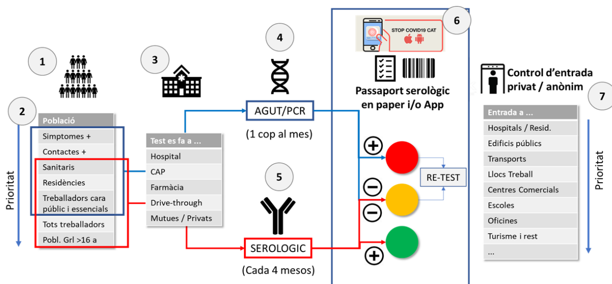
Figura 4. Esquema general de cribratge, diagnòstic i establiment d'una acreditació d'immunitat indicativa de l'estat infectiu de l'individu.
